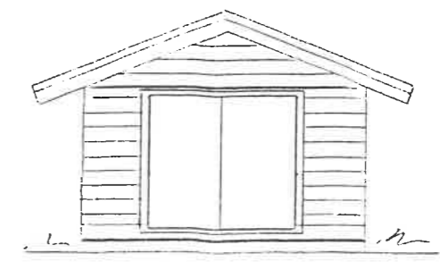
FASAD VÄSTER
