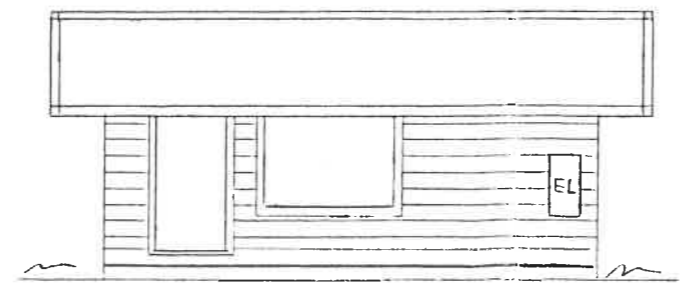
FASAD NORR
