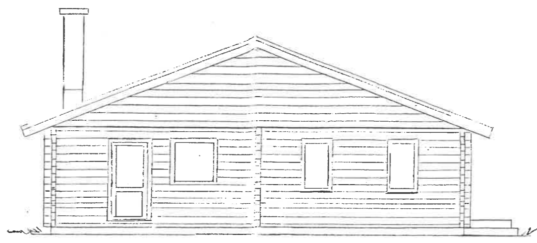
FASAD SÖDER
