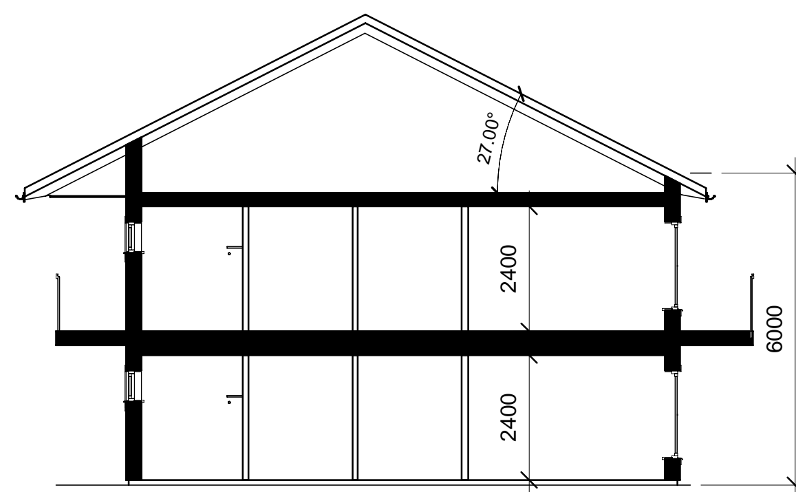
1 SEKTION HUS 3 OCH 4 1:100
